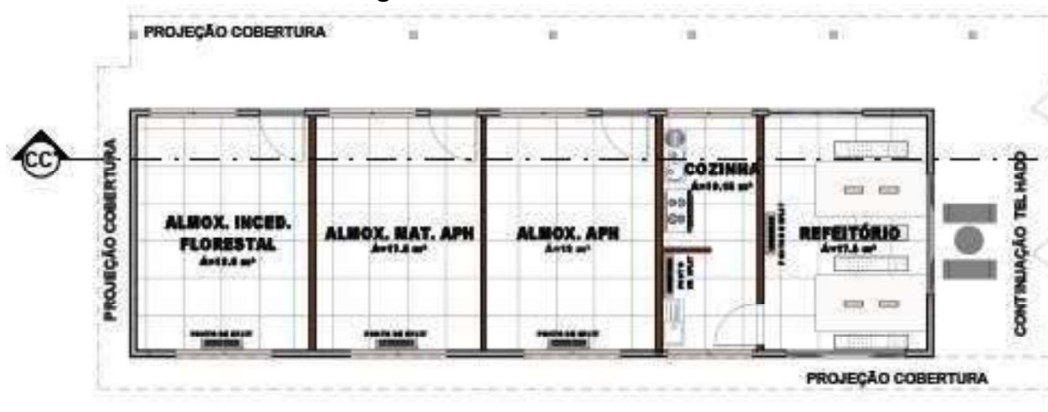
Figura 03 – BLOCO ALMOXARIFADO
