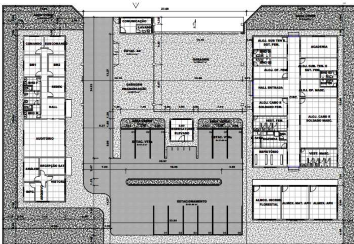
Figura 01 – PLANTA DE LOCAÇÃO.
